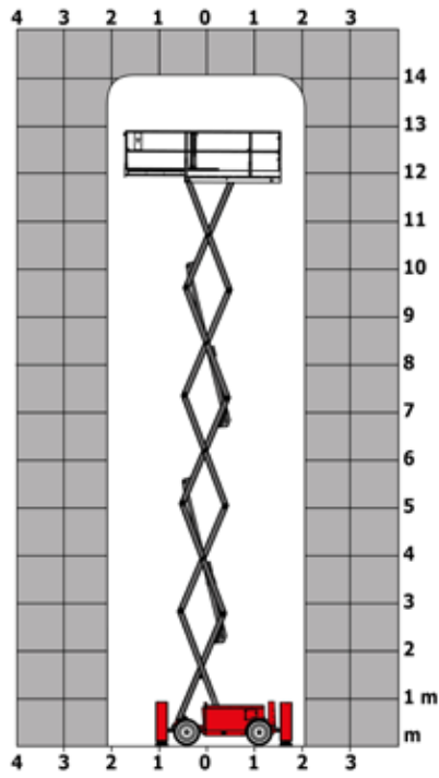
Gráfico da carga para plataforma elevatória (métrico)
